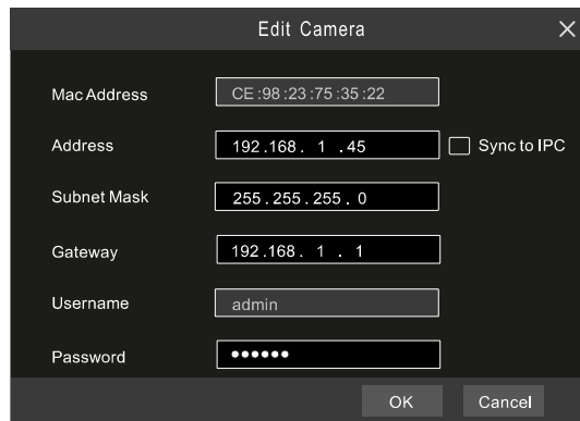
Рис. 1.5. Меню редактирования настроек IP-видеокамеры
