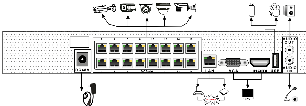
Рис. 1.1. Задняя панель LTV RNE-161 0G
