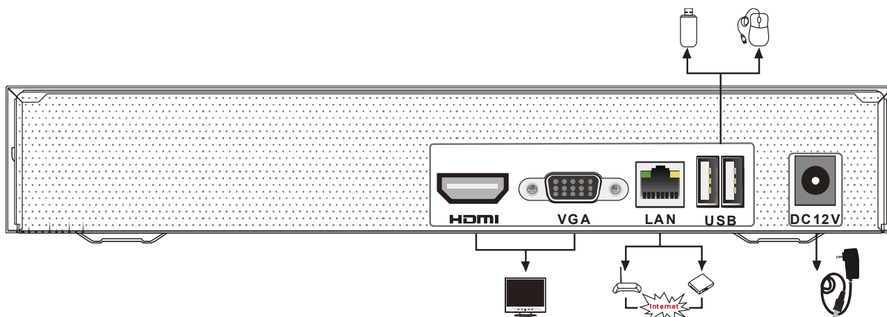
Рис. 1.1. Задняя панель IP-видеорегистратора
