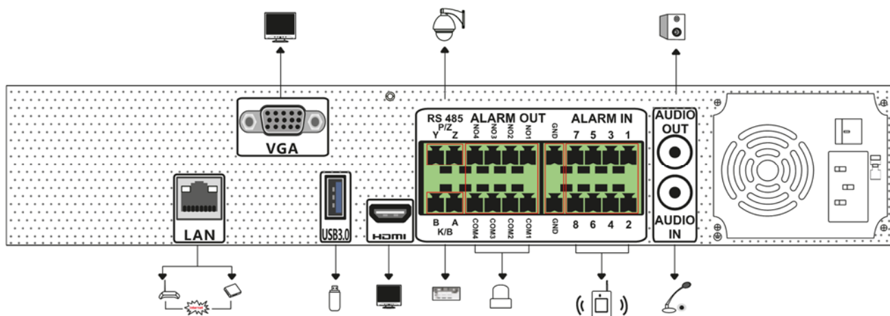
Рис. 1.1. Задняя панель LTV RNE-320 01 FR
