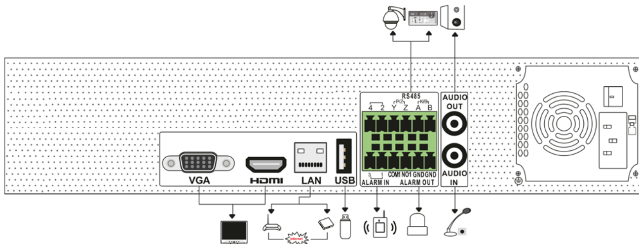
Рис. 1.1. Задняя панель LTV RNE-321 01
