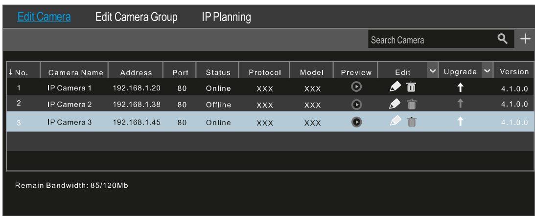
Рис. 1.6. Меню редактирования списка IP-видеокамер
