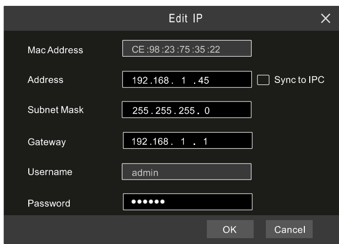
Рис. 1.5. Меню редактирования настроек IP-видеокамеры
