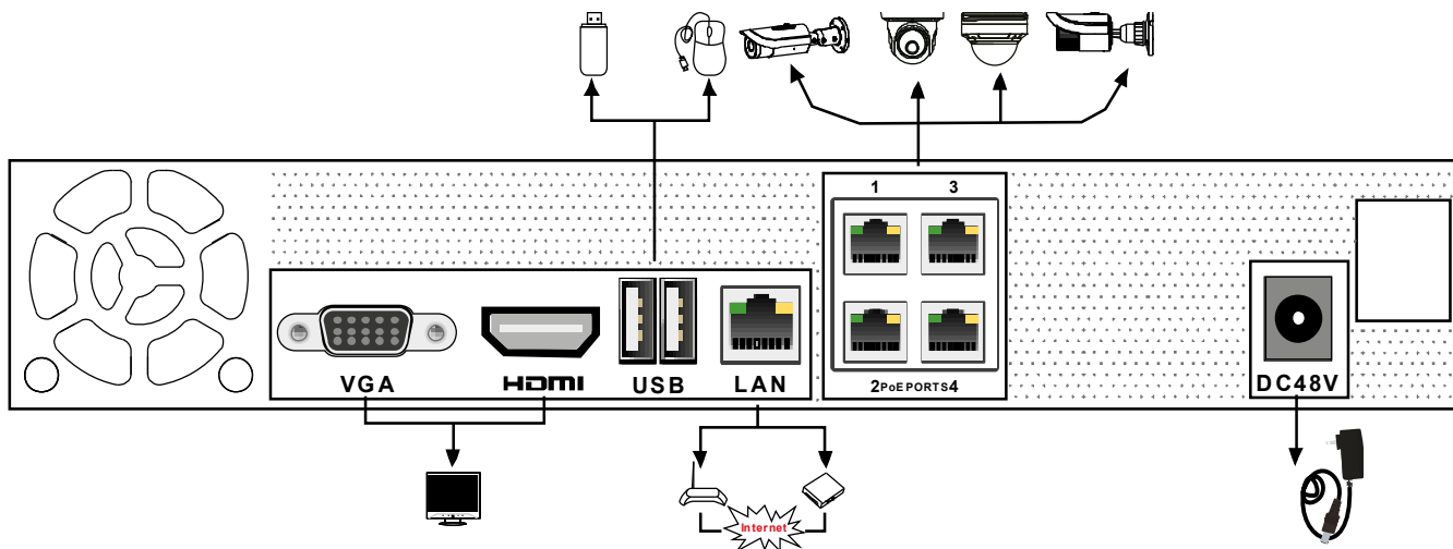
Рис. 1.1. Задняя панель LTV RNE-041 0G
