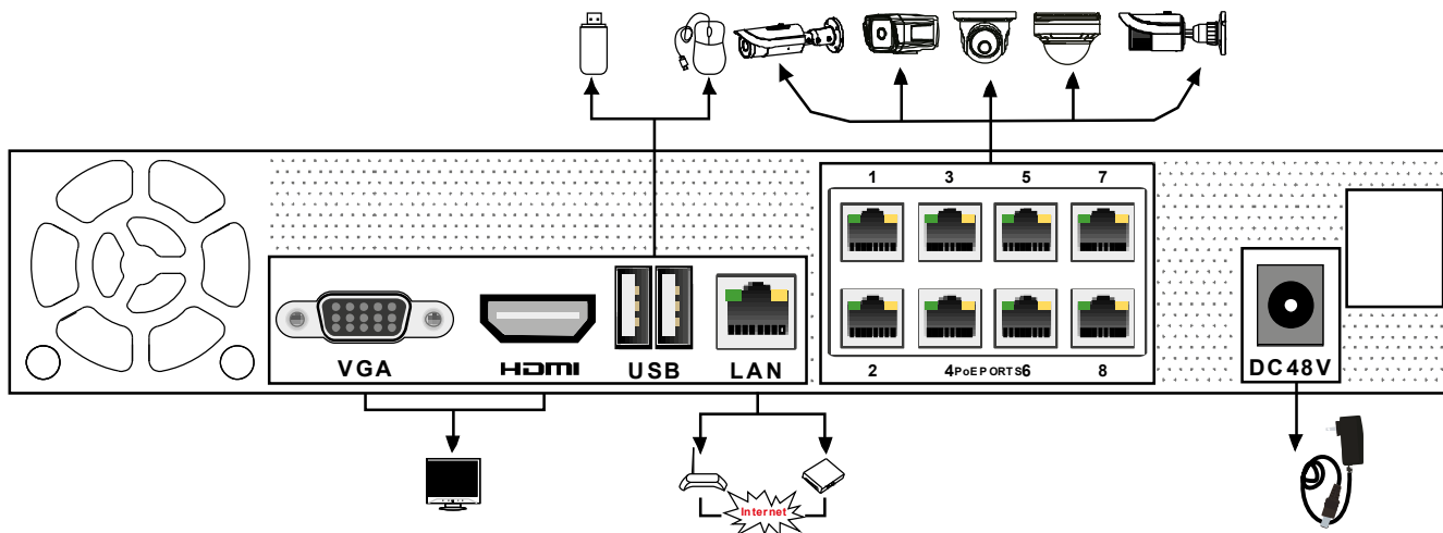
Рис. 1.2. Задняя панель LTV RNE-081 0G
