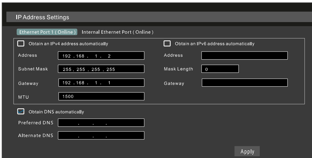
Рис. 1.4. Меню настроек TCP/IP
