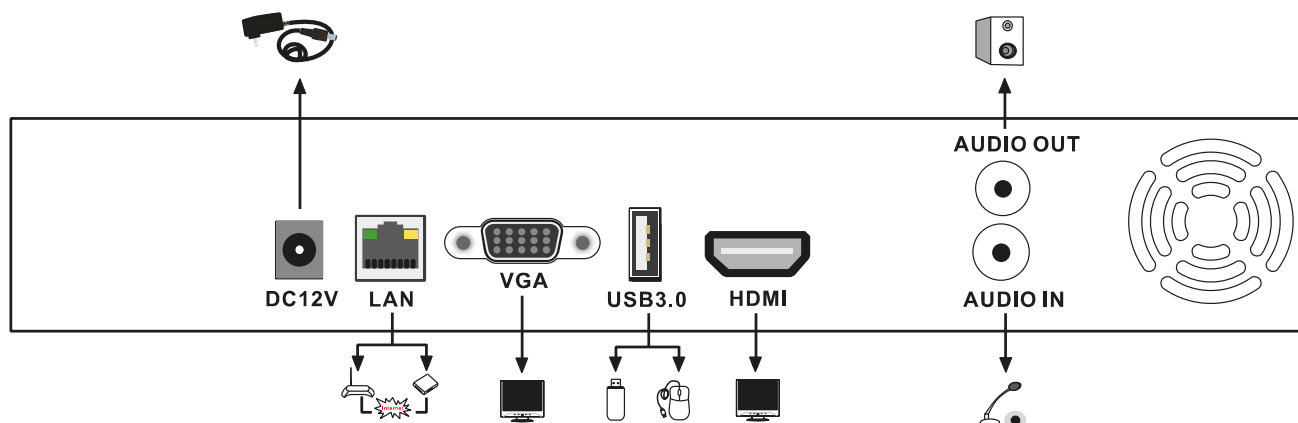
Рис. 1.1. Задняя панель LTV RNE-160 00 FR
