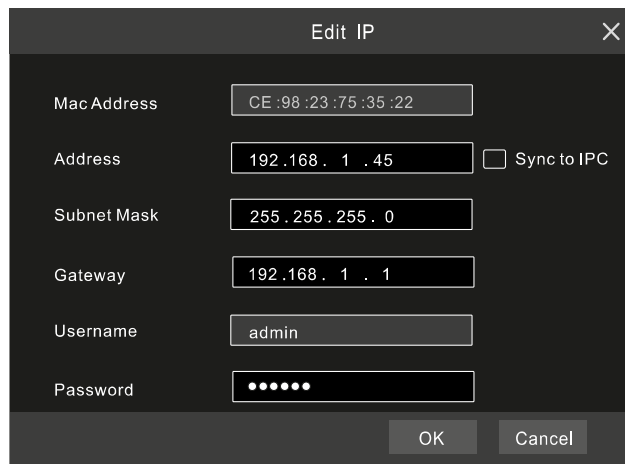
Рис. 1.5. Меню редактирования настроек IP-видеокамеры
