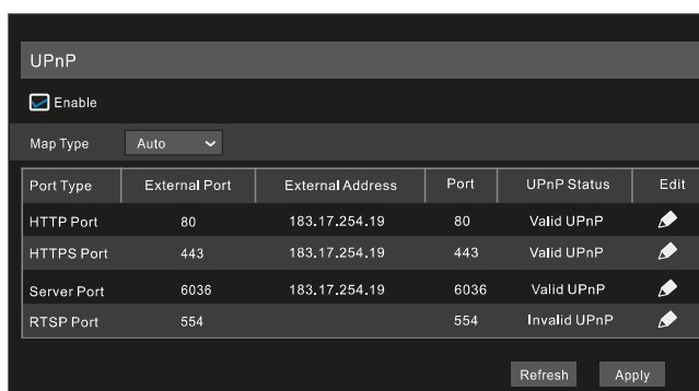
Рис. 1.8. Настройки протокола UPnP
